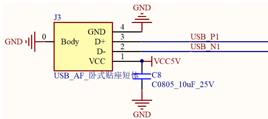
图 2-5 U 盘参考电路
