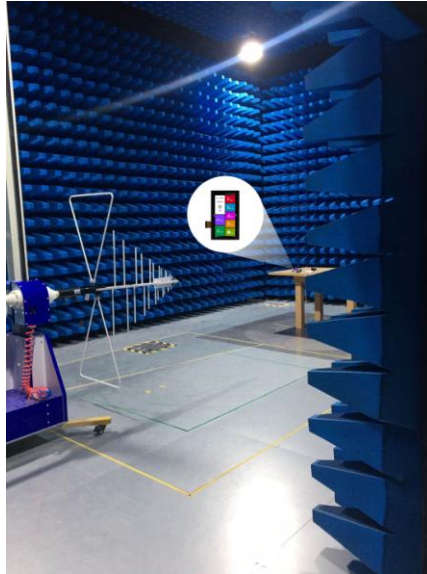
图 5-4 RE 测试图
