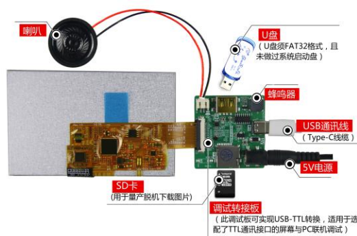
图 1-5 调试工具图
