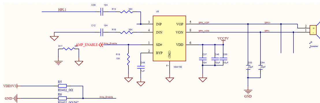
图 2-3 音频参考电路
