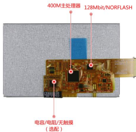
图 1-4 硬件配置图
