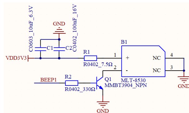
图 2-4 蜂鸣器参考电路
