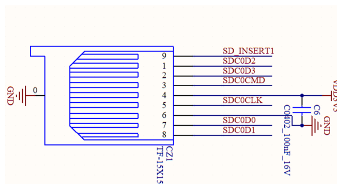
图 2-2 SD 卡参考电路
